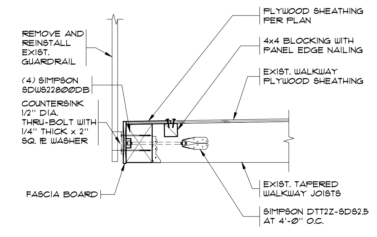
SECTION 4 SCALE: 3/4" = 1'-0"
