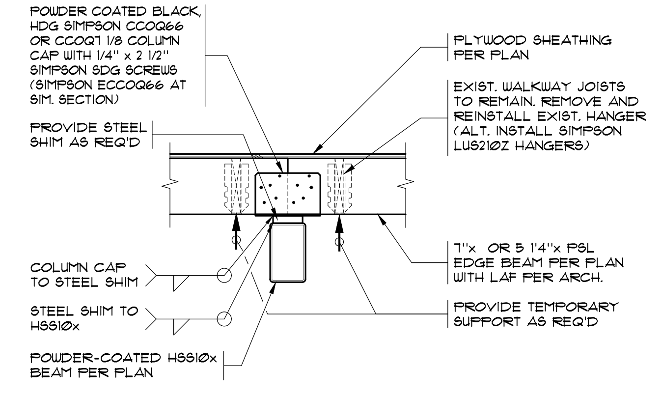
SECTION 2 SCALE: 3/4" = 1'-0"
