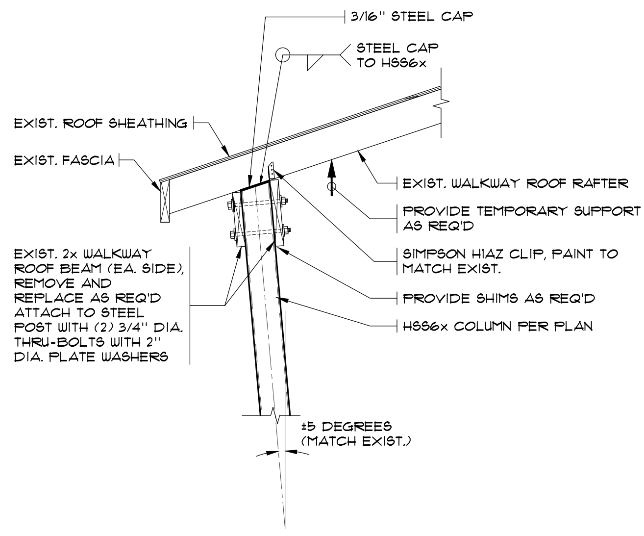
SECTION 1 SCALE: 3/4" = 1'-0"
