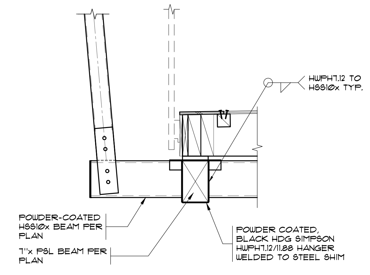
SECTION 6 SCALE: 3/4" = 1'-0"
