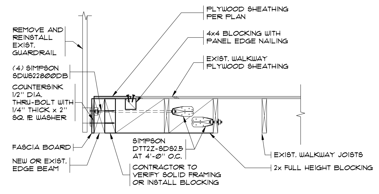
SECTION 3 SCALE: 3/4" = 1'-0"
