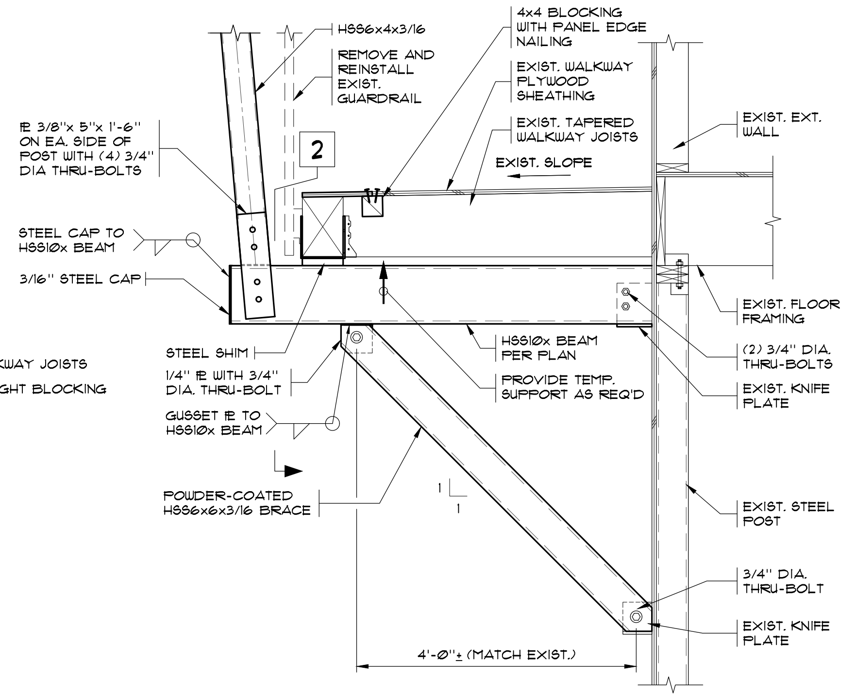
SECTION 8 SCALE: 3/4" = 1'-0"
