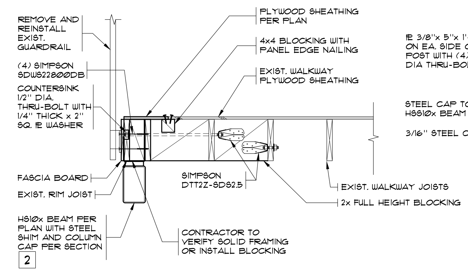
SECTION 7 SCALE: 3/4" = 1'-0"
