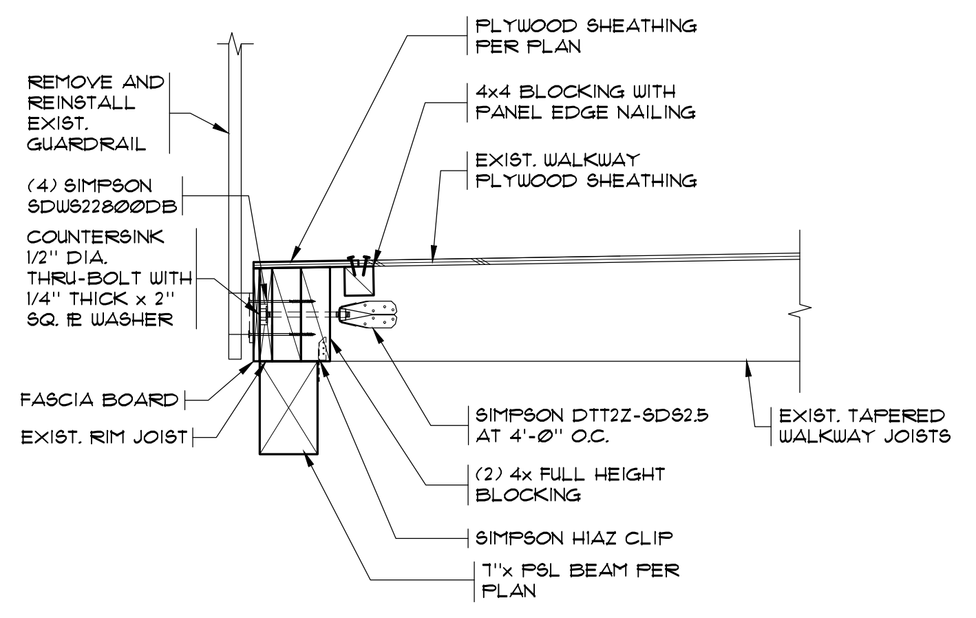
SECTION 5 SCALE: 3/4" = 1'-0"
