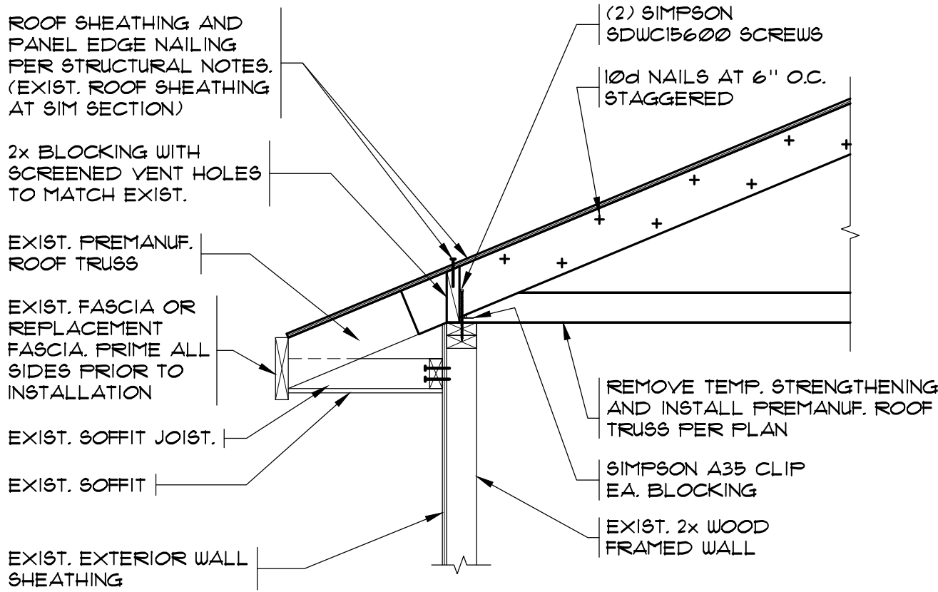
SECTION 1 SCALE: 3/4" = 1'-0"
